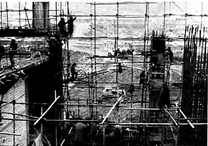
Nga puna për ndërtimin e montimin në kantieret e hidrocentralit „Enver Hoxha” në Koman
