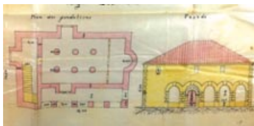
Σχέδιο 13: Στράτσιανν – Εκκλησία Αγία Παρασκευή.
