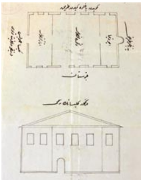
Σχέδιο 46: Ελληνική εκκλησία Κόνιτσας.
