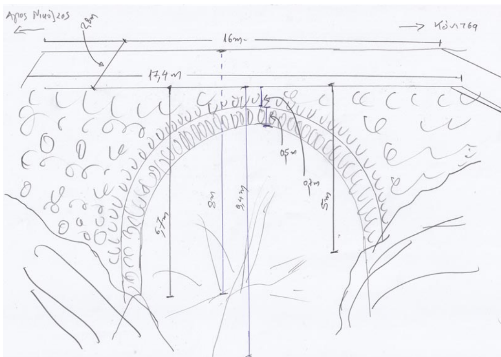
Σχέδιο 1. Απεικόνιση της γέφυρας εκ των κατόντων.
